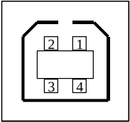
USB「B」型插头接口
